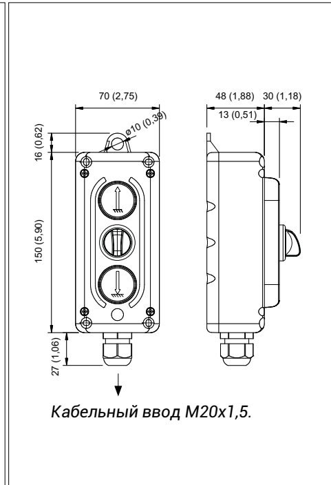
ТЕХНИЧЕСКИЙ ЧЕРТЕЖ – TLP3.D
