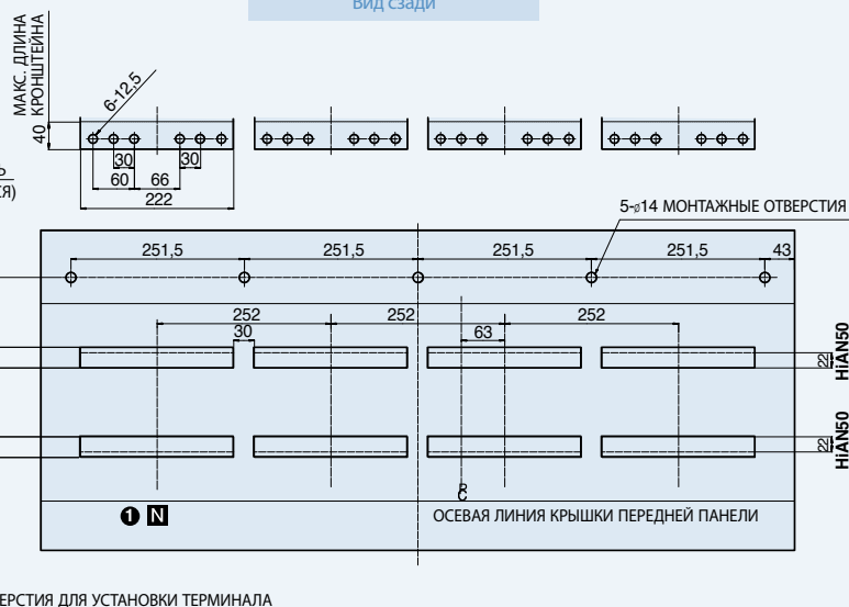
Вид сзади
