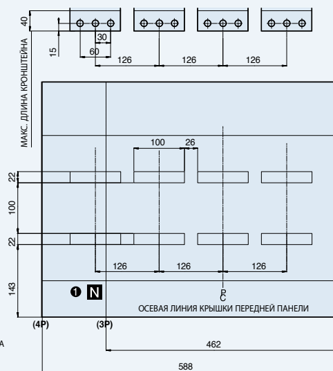
Вид сзади
