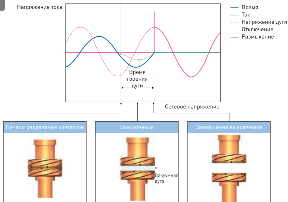
Диаграмма отключения
