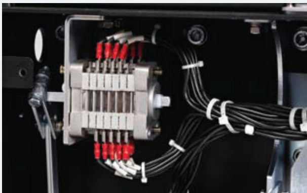
Вспомогательный переключатель
