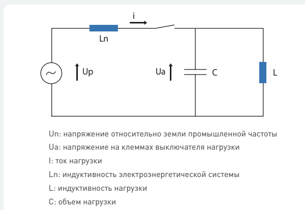
[Рис. 2] Однофазная схема замещения для отключения индуктивного тока
