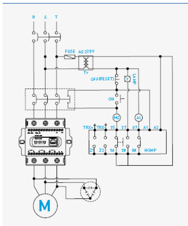
Трёхфазная схема (вспом. клеммы: предупреждение макс. тока)
