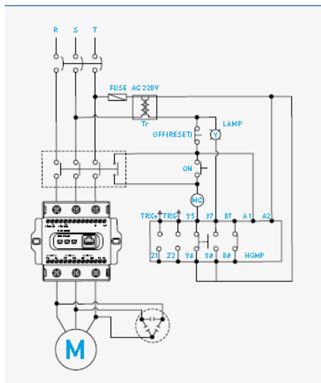
Трёхфазная схема (вспом. клеммы: мгновенная защита)
