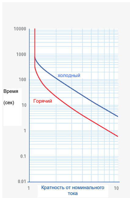
Обратная задержка, класс 10
