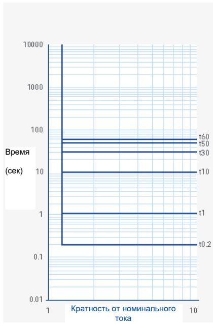
Независимая задержка
