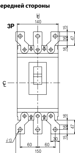
Подключение с передней стороны
