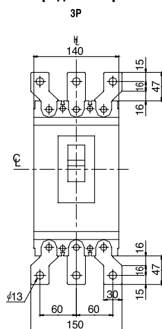
Схема сверления
