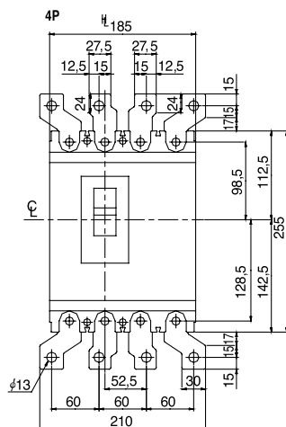
Установочные отверстия в панели
