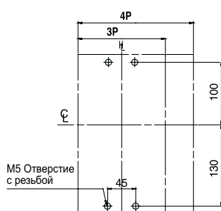
Схема сверления
