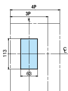
Установочные отверстия в панели
